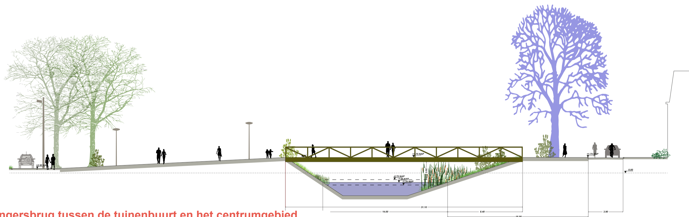
principe voetgangersbrug tussen de tuinenbuurt en het centrumgebied
