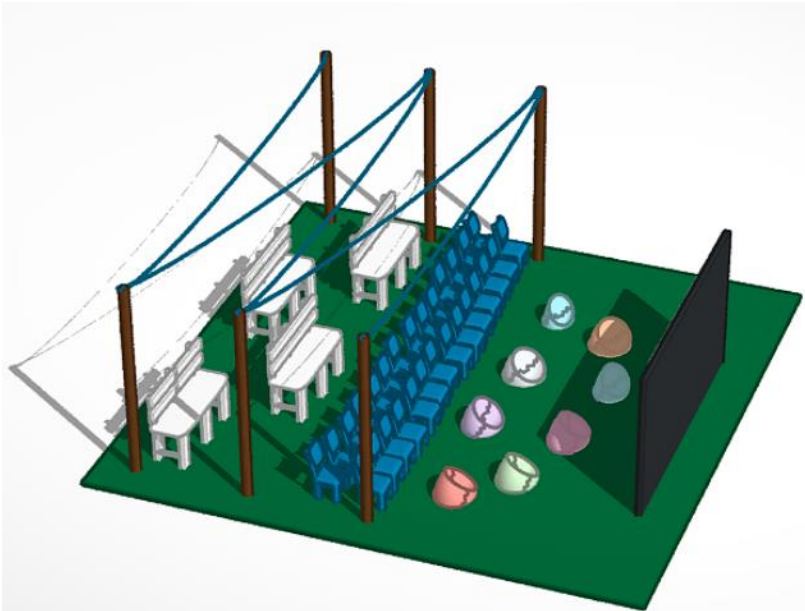
Figuur 7.2, Het 3D ontwerp van de buitenbioscoop.
