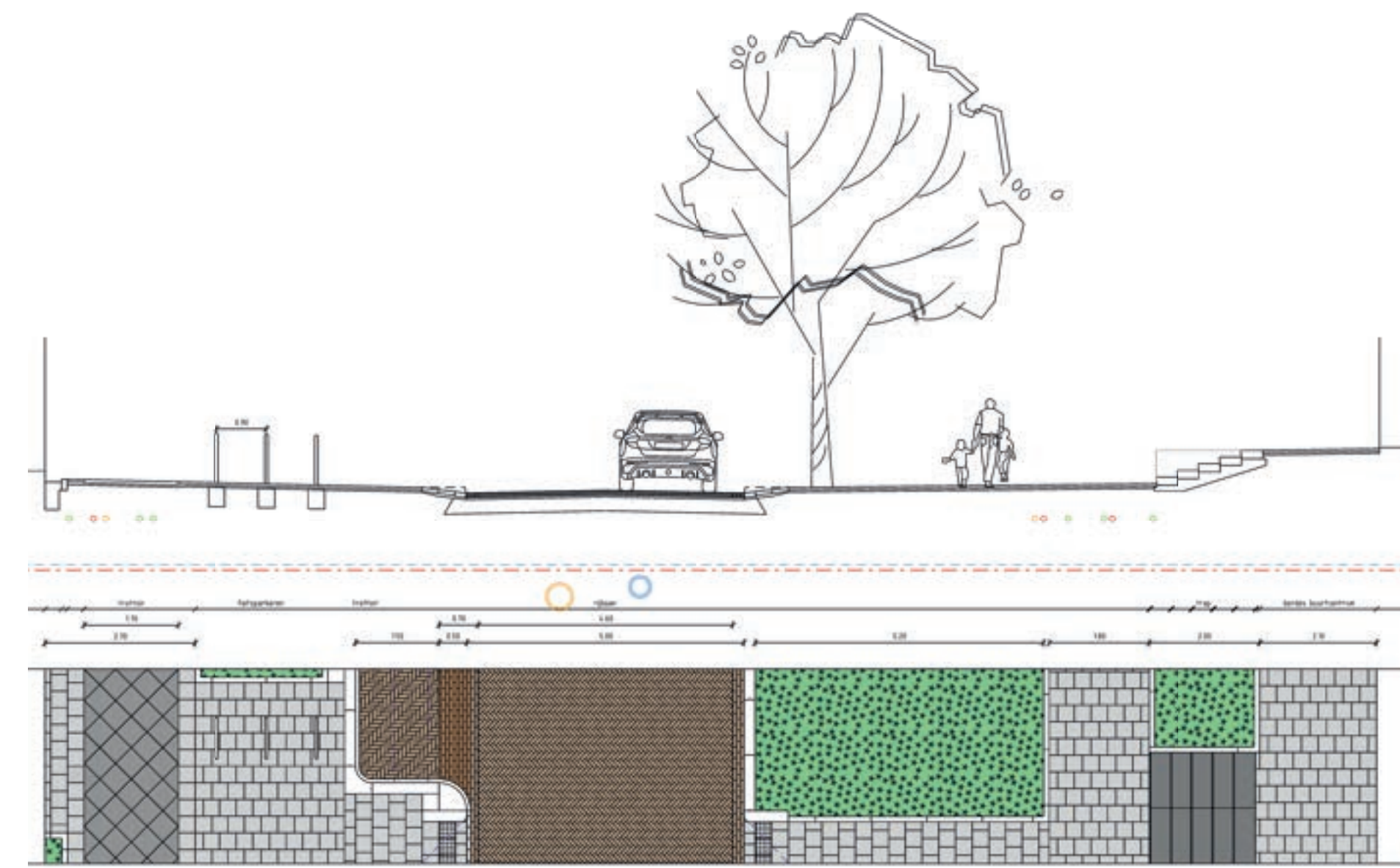
profiel C-C' Samuel Mullerstraat
