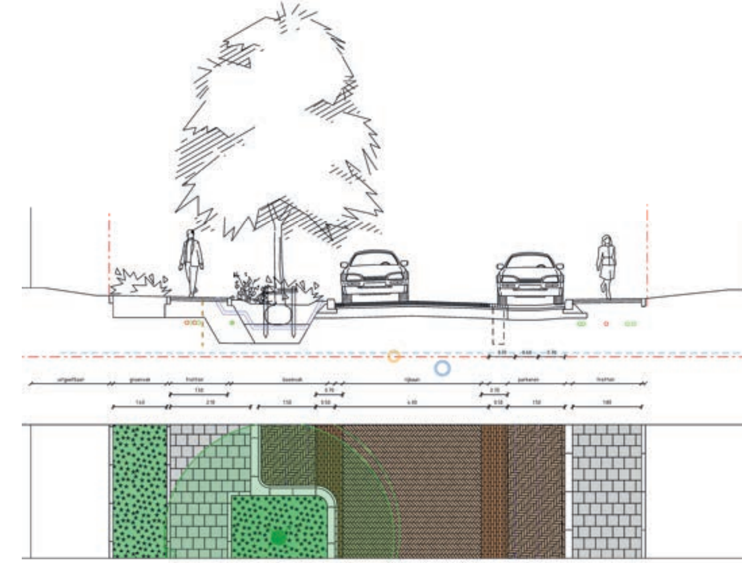
profiel E-E' Slotemaker de Bruinestraat
