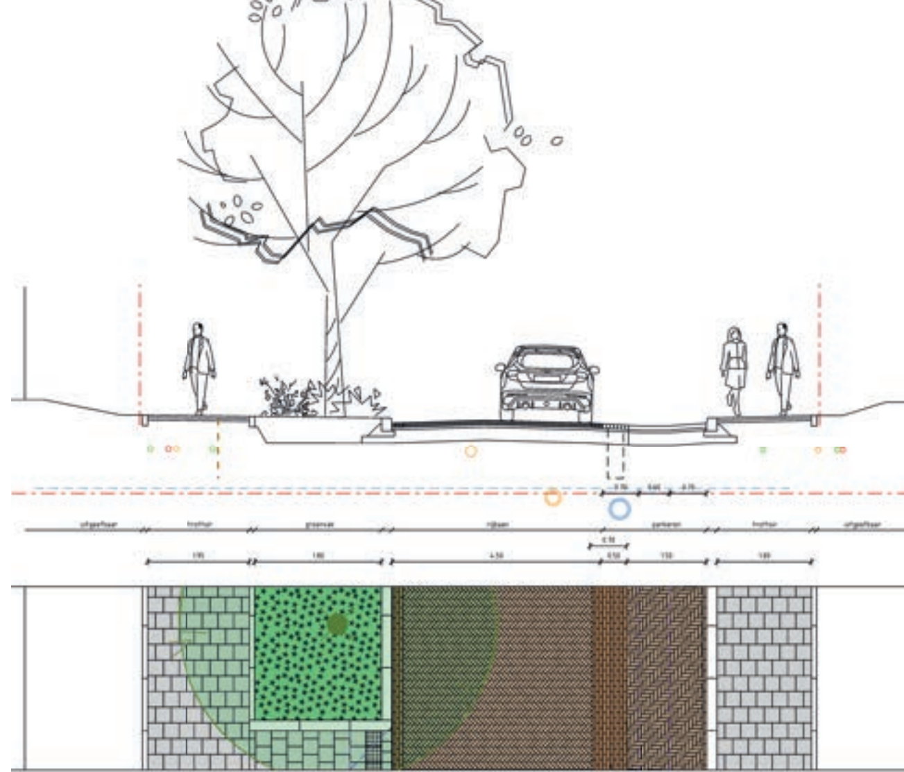
profiel D-D' Nolenslaan
