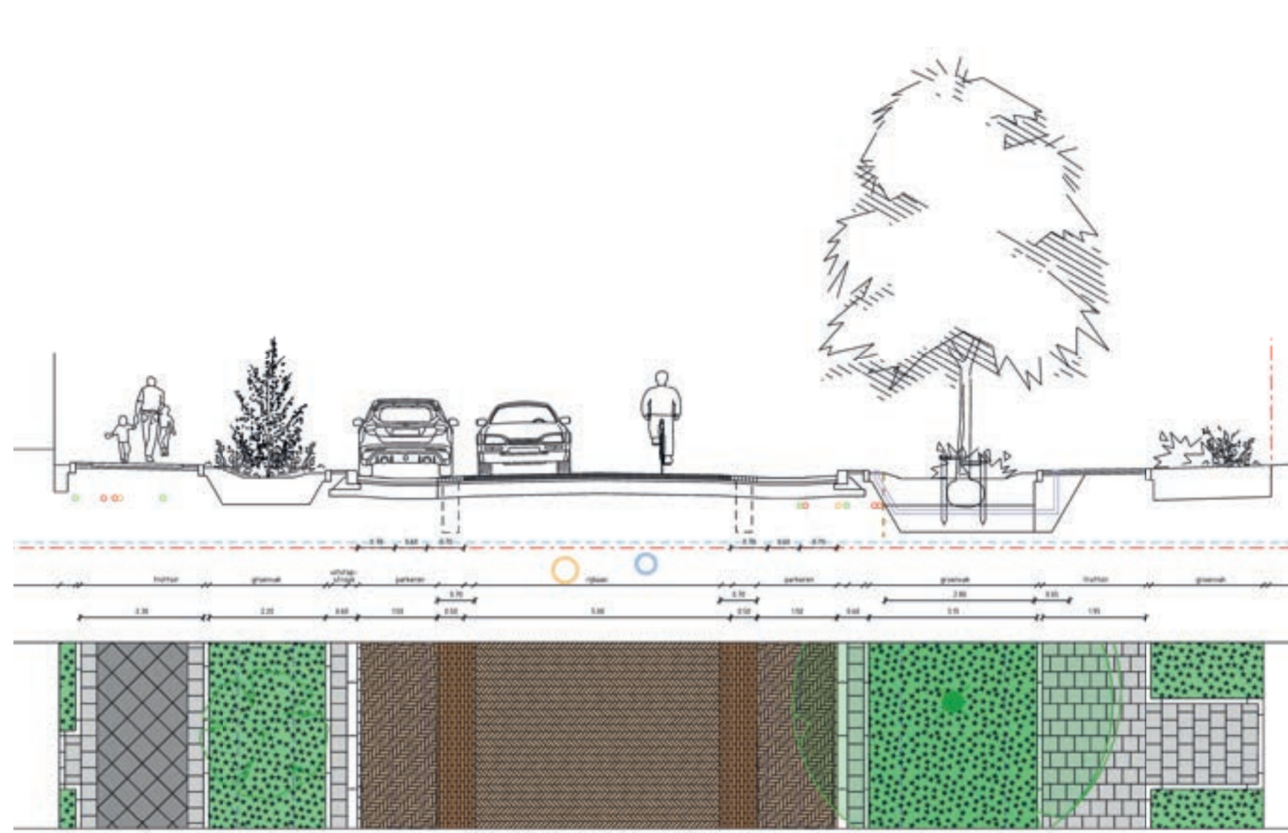
profiel E-E' Slotemaker de Bruinestraat
