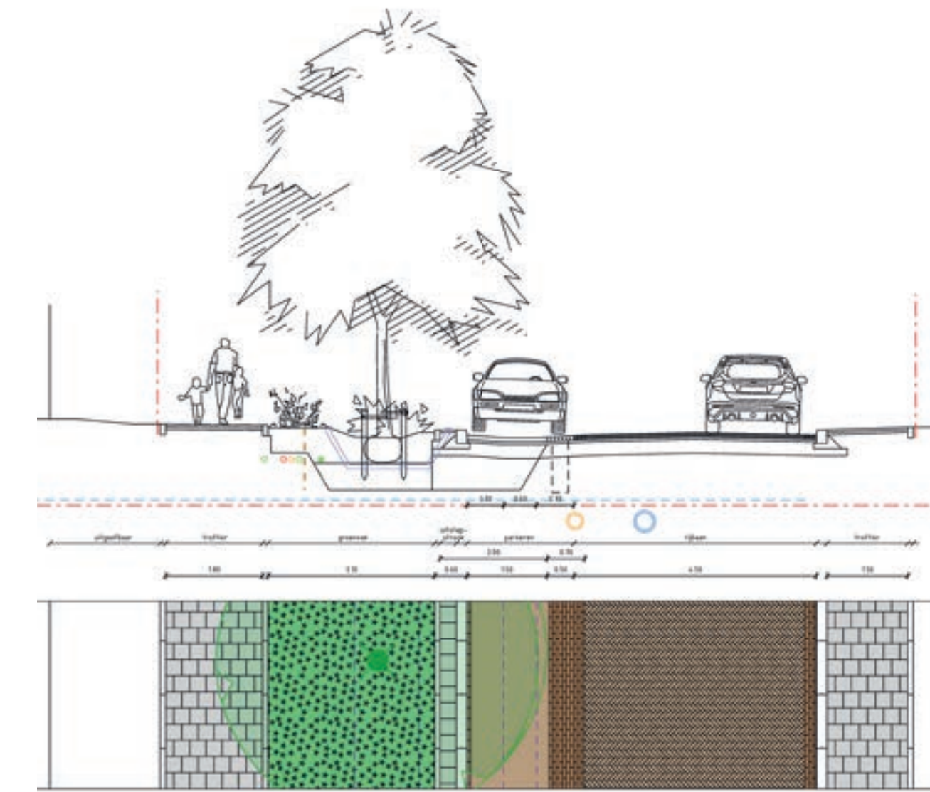
profiel C-C' Samuel Mullerstraat
